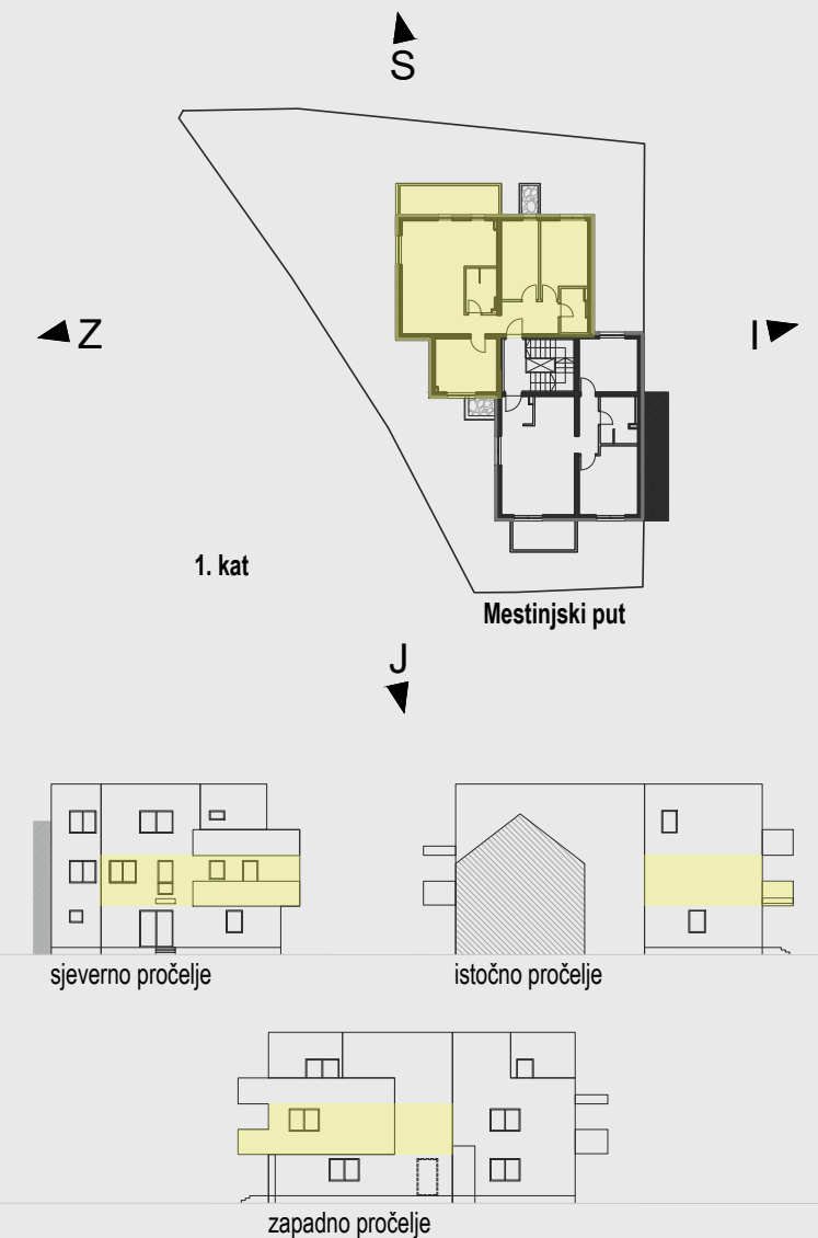
ČETVEROSOBNI STAN_1. KAT_STAN A1
